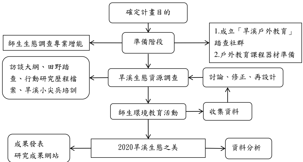
圖1.研究流程圖
